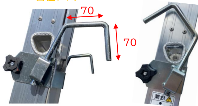
自在式滑り止め端具
